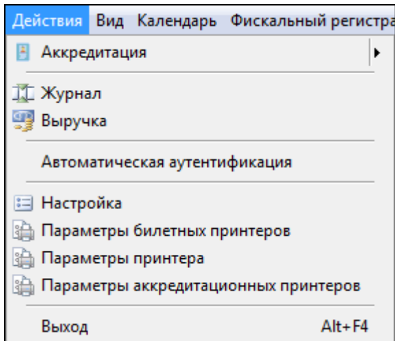
Рис.3.5. Меню «Действия»
